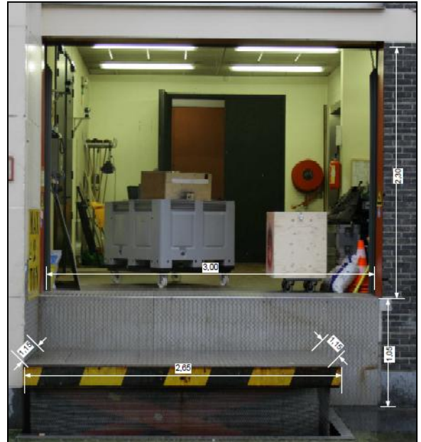
Afmetingen loskade
