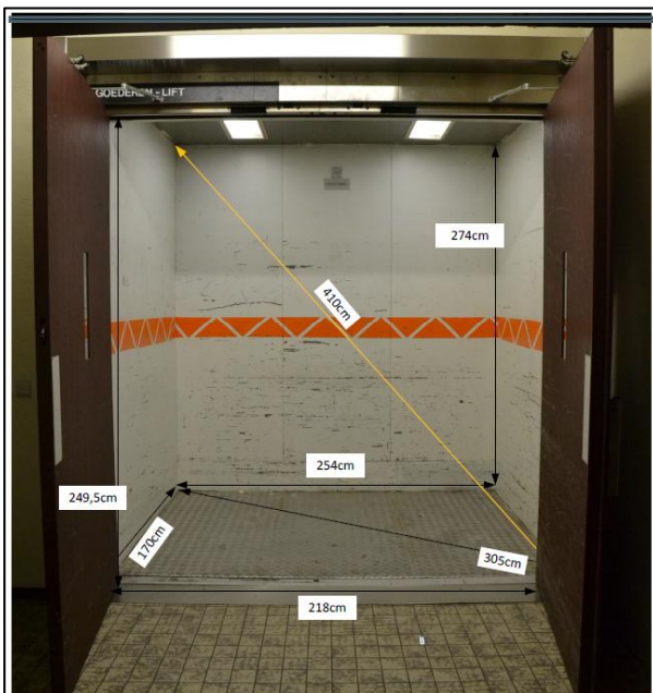
Afmetingen lift voor kleine zaal
